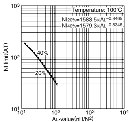
NI limit vs. AL 值(代表例) PC95EPC10 磁心(带空隙)
