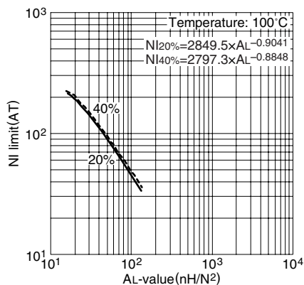
NI limit vs. AL 值(代表例) PC95EPC13 磁心(带空隙)
