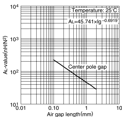
AL 值 vs. 气隙长度(代表例) PC95EPC19 磁心
