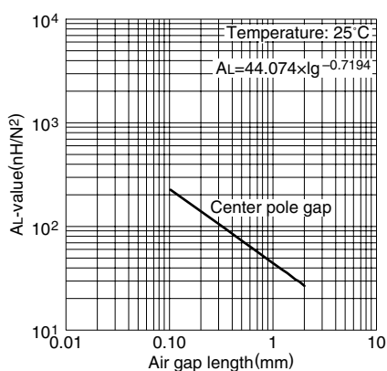
AL 值 vs. 气隙长度(代表例) PC95EPC17 磁心
