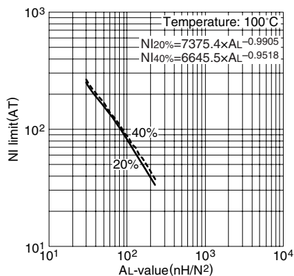
NI limit vs. AL 值(代表例) PC95EPC19 磁心(带空隙)
