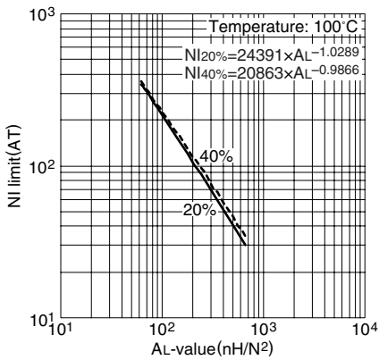
NI limit vs. AL 值(代表例) PC47LP22/13 磁心(带空隙)
