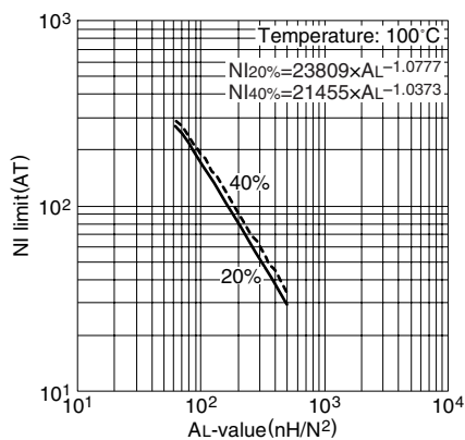
NI limit vs. AL 值(代表例) PC95EPC27 磁心(带空隙)
