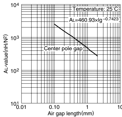
AL 值 vs. 气隙长度(代表例) PC47PQ50/50 磁心
