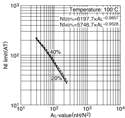
NI limit vs. AL 值(代表例) PC95EPC17 磁心(带空隙)
