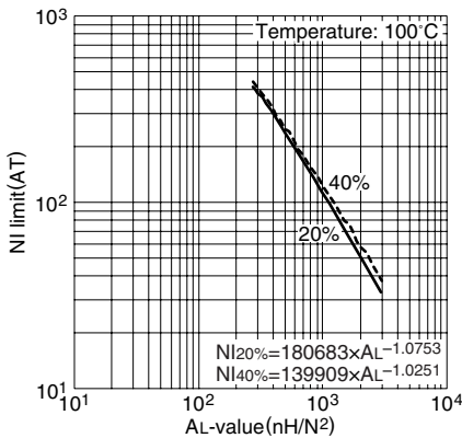
NI limit vs. AL 值(代表例) PC47PQ50/50 磁心(带空隙)
