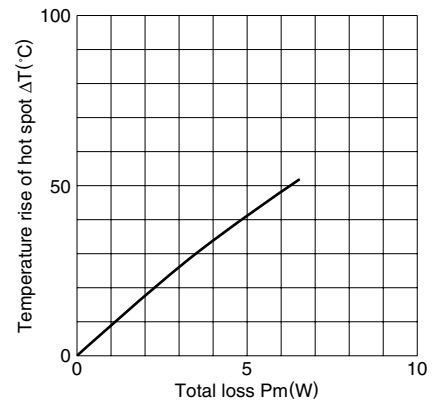
温度上升 vs. 总损耗特性(代表例) PQ50/50 磁心
