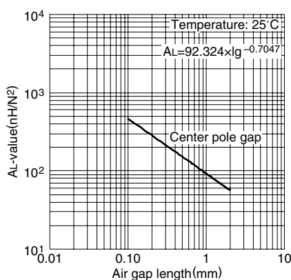
AL 值 vs. 气隙长度(代表例) PC95EPC27 磁心
