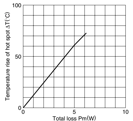
温度上升 vs. 总损耗特性(代表例) PQ40/40 磁心
