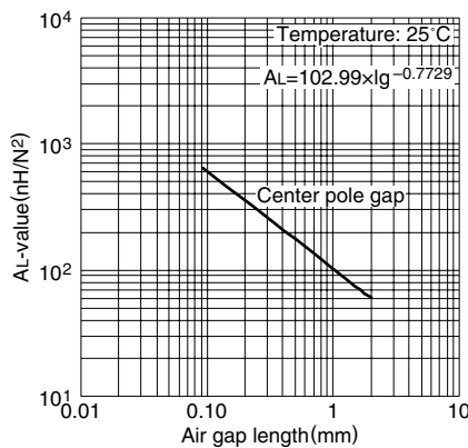
AL 值 vs. 气隙长度(代表例) PC47LP22/13 磁心
