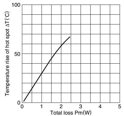
温度上升 vs. 总损耗特性(代表例) LP22/13 磁心
