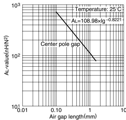
AL 值 vs. 气隙长度(代表例) PC95PQI20/9 磁心
