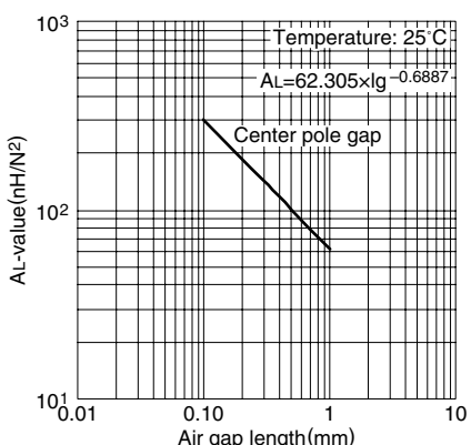
AL 值 vs. 气隙长度(代表例) PC95EIR18/5/12 磁心
