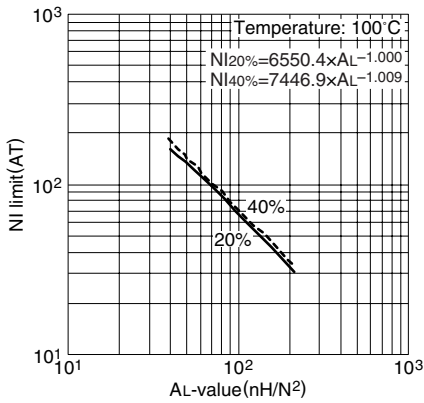
NI limit vs. AL 值(代表例) PC95EL11X4 磁心(带空隙)
