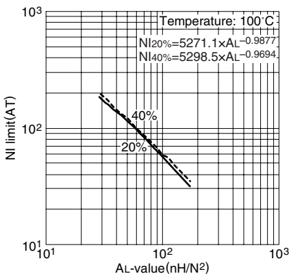
NI limit vs. AL 值(代表例) PC95EI14/5/5 磁心(带空隙)
