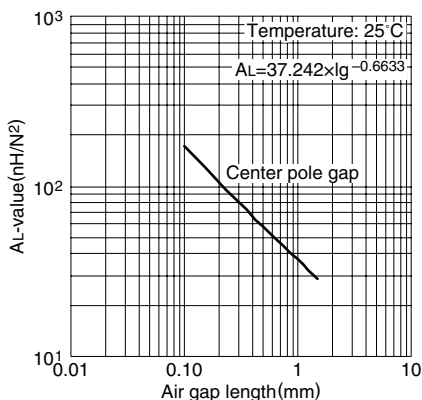
AL 值 vs. 气隙长度(代表例) PC95EI14/5/5 磁心
