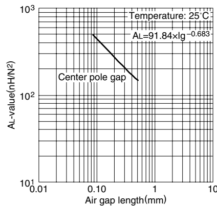
AL 值 vs. 气隙长度(代表例) PC95ELT15.5X4.3 磁心
