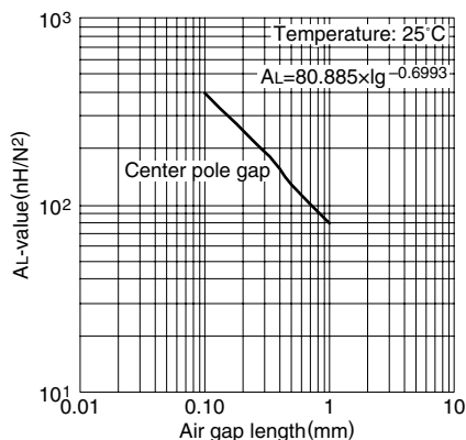
AL 值 vs. 气隙长度(代表例) PC95PQI16/7.8 磁心
