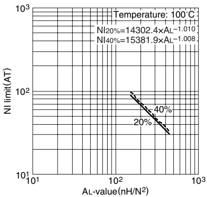
NI limit vs. AL 值(代表例) PC95ELT15.5X4.3 磁心(带空隙)
