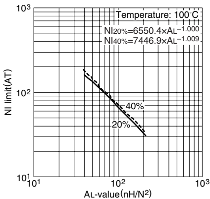
NI limit vs. AL 值(代表例) PC95EL13X4.4 磁心(带空隙)
