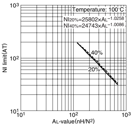
NI limit vs. AL 值(代表例) PC95PQI20/9 磁心(带空隙)
