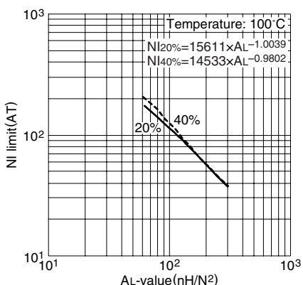
NI limit vs. AL 值(代表例) PC95EIR18/5/12 磁心(带空隙)
