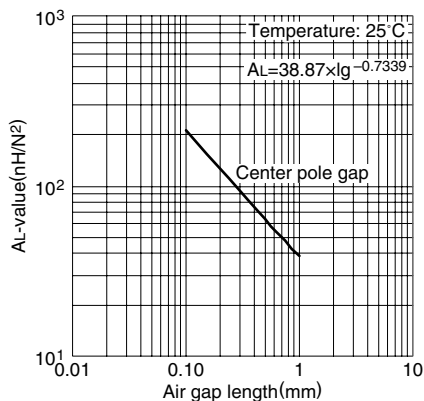
AL 值 vs. 气隙长度(代表例) PC95EL11X4 磁心
