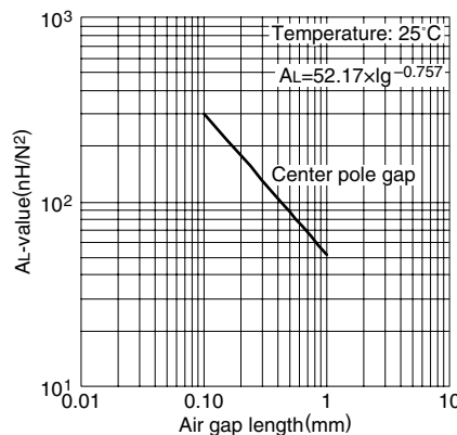
AL 值 vs. 气隙长度(代表例) PC95EL13X4.4 磁心
