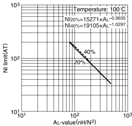
NI limit vs. AL 值(代表例) PC95PQI16/7.8 磁心(带空隙)
